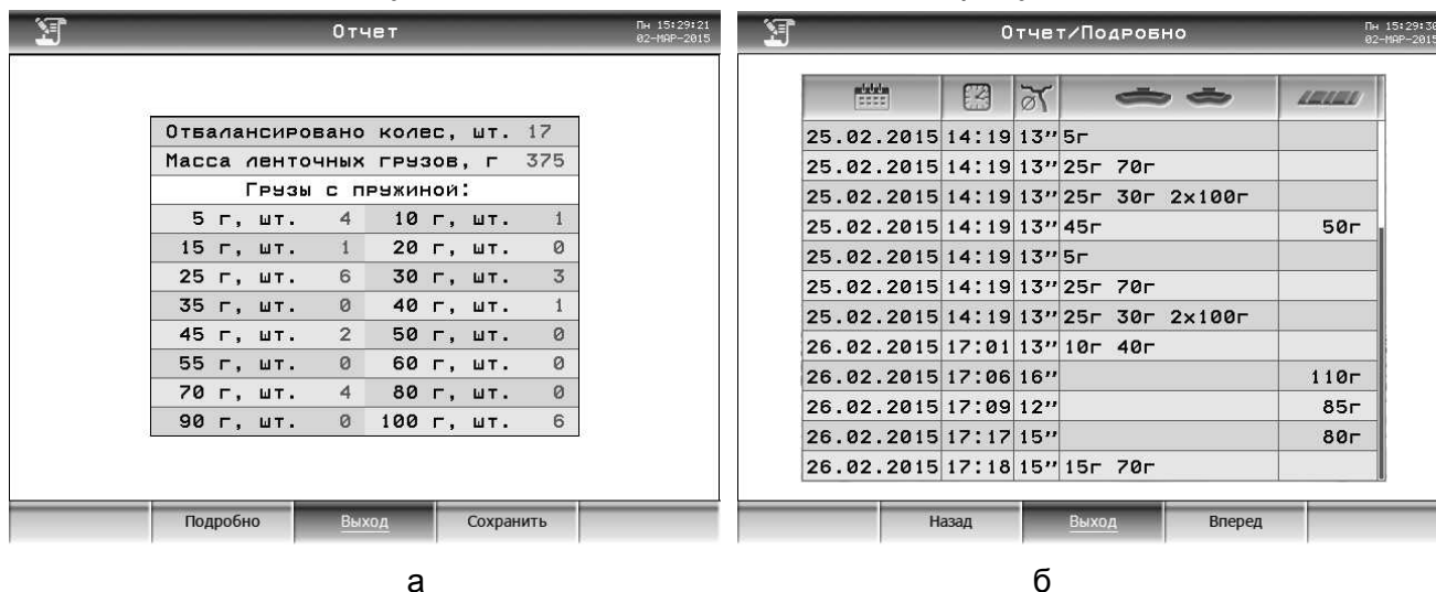
Рисунок 7.7 - Отчет
