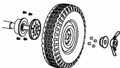
д – установка на фланец
