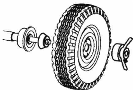
а – конус изнутри
