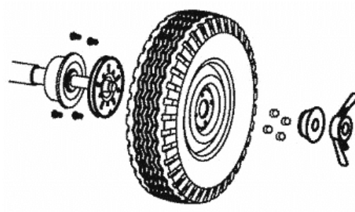
Рисунок 5.4 - Установка на фланец
