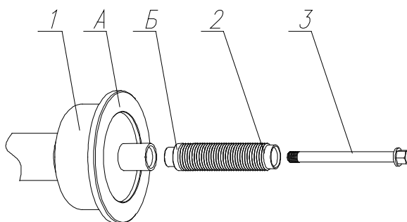
а – сборка вала
