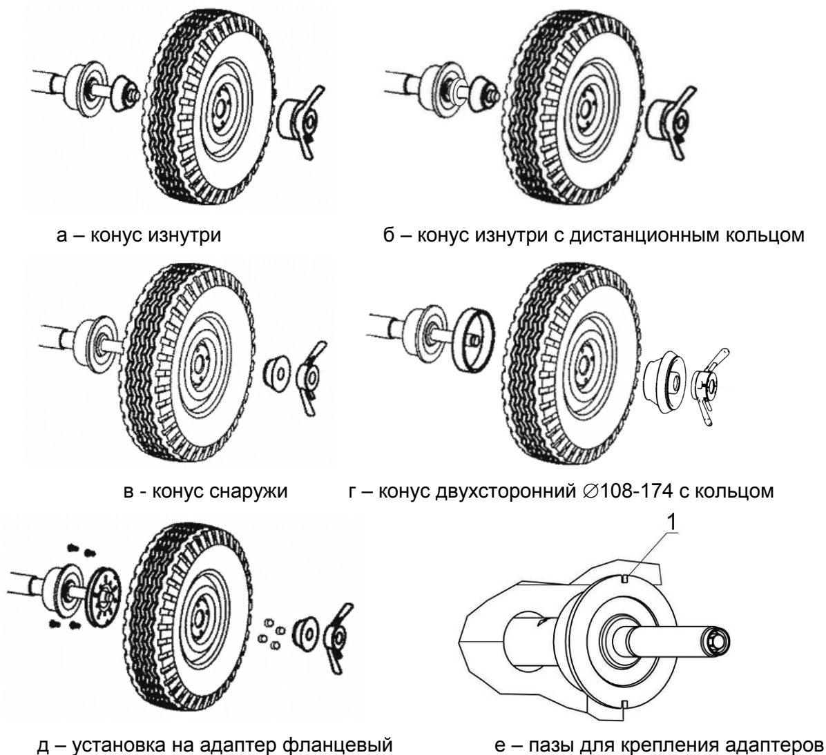
Рисунок 5.1 – Установка колеса
