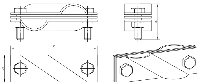
Рисунок 1 – Габаритные размеры
