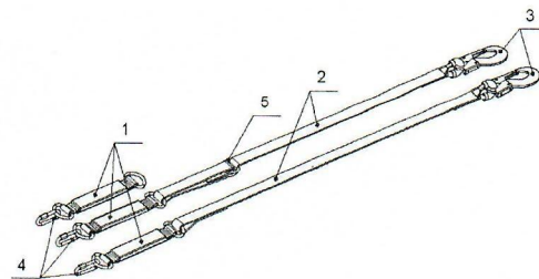
Рис.1 Схематическое изображение страховочного стропа и амортизатора «а»
