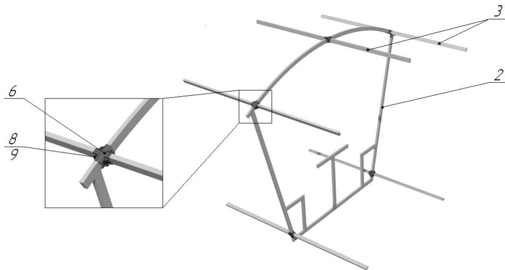
Рис.2 Сборка внутреннего каркаса
