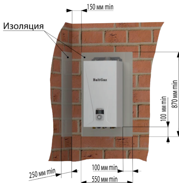
Рис. 6 Монтаж котла
