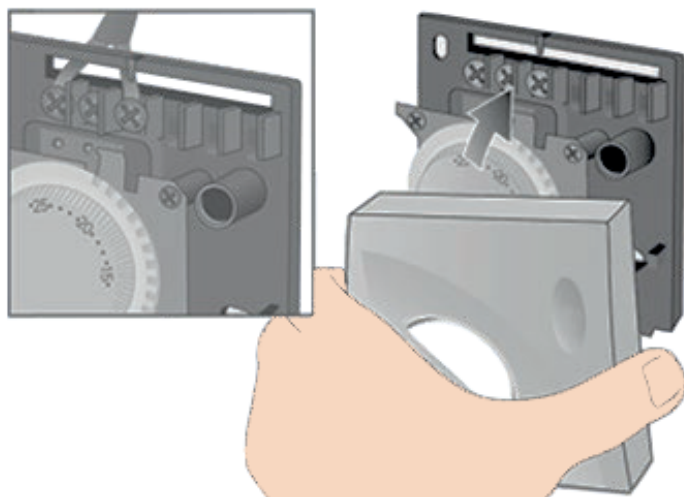
Рис. 3 Подключение соединительного кабеля к комнатному термостату
