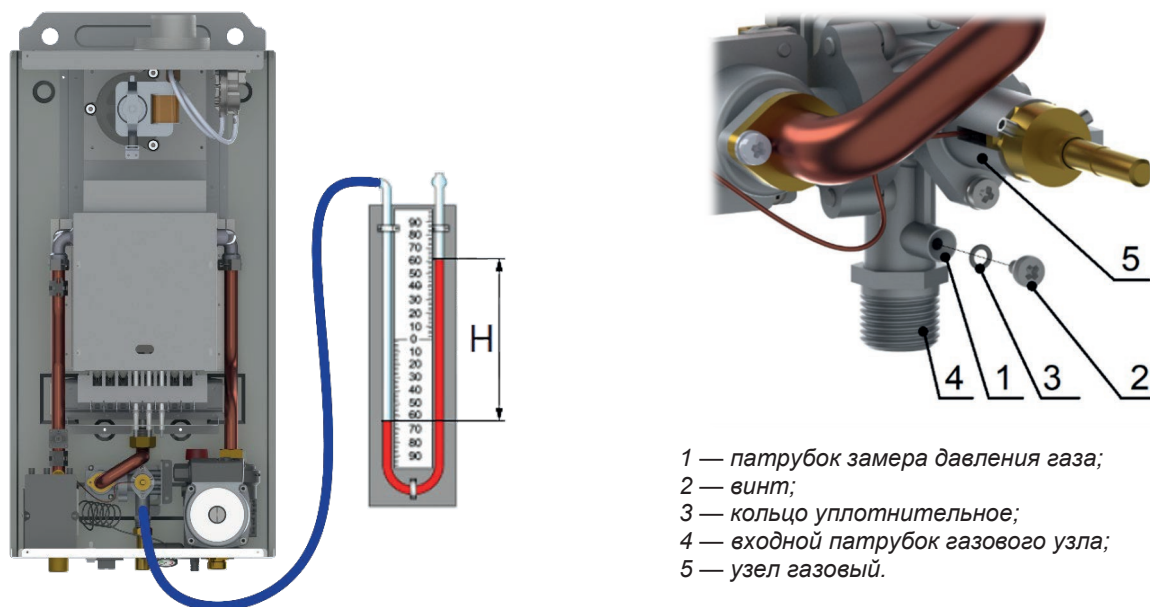
Рис. 12 Подключение дифманометра
