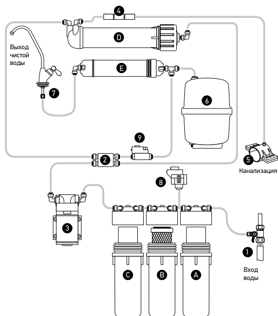
Рис.2. Принципиальная схема подключения фильтра Start Osmos.
