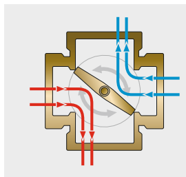
Схема работы четырёхходового клапана в режиме полного закрытия
