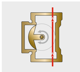
Схема работы четырёхходового клапана в смесительном режиме полуоткрытия (рабочий режим)
