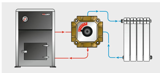
Схема работы четырёхходового клапана в режиме полного закрытия
