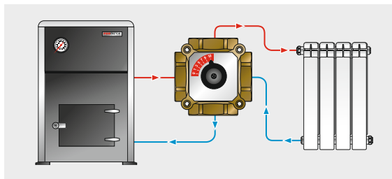
Схема работы четырёхходового клапана в режиме полного открытия
