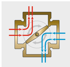
Схема работы четырёхходового клапана в режиме полного открытия
