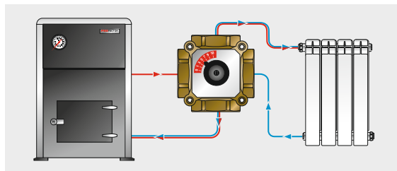
Схема работы четырёхходового клапана в смесительном режиме полуоткрытия (рабочий режим)
