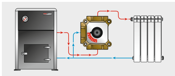
Схема работы трёхходового клапана в режиме полного открытия
