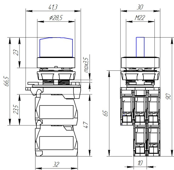
Рис.10. Переключатель с рукояткой.
