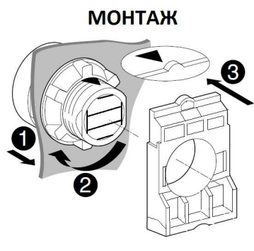
Рис.13 Монтаж и демонтаж выключателя.
