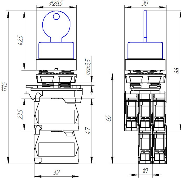
Рис.11. Переключатель с ключом.
