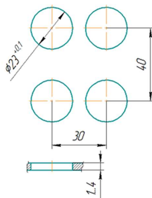
Рис.1 Монтажные размеры
