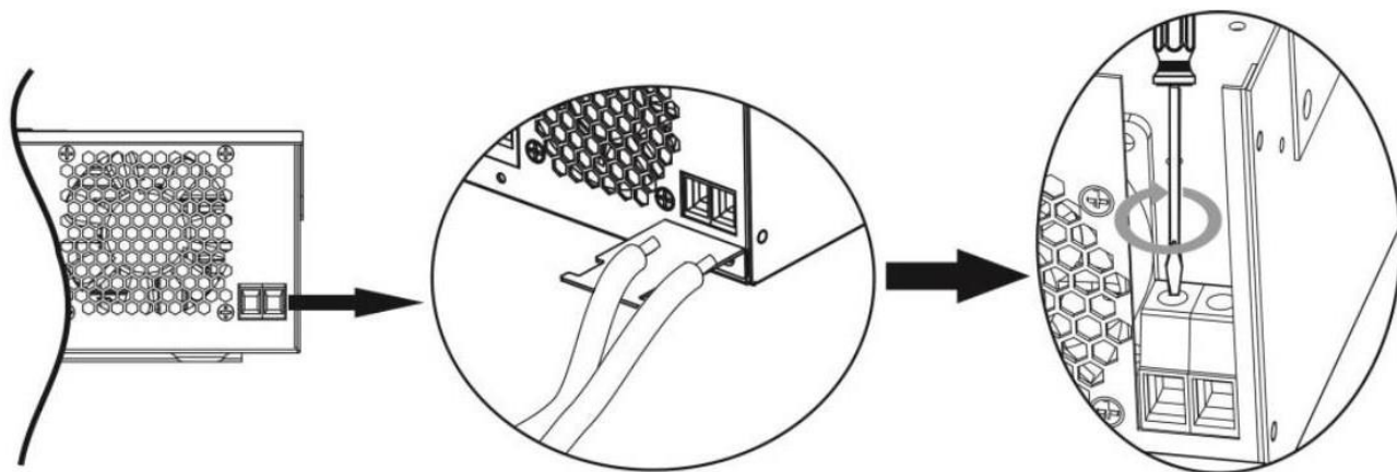
Рисунок 5.12 Подключение PVBox к инвертору.
