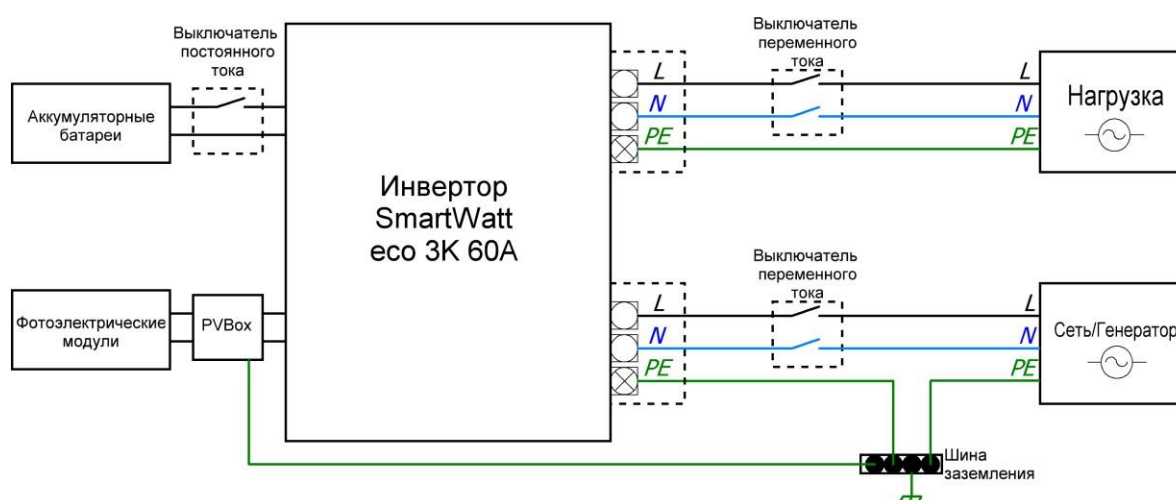
Рисунок 3.1 Структурная схема подключения фотоэлектрической системы.
