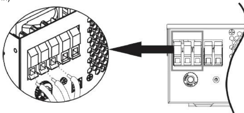
Рисунок 5.6 Подключение проводов входа переменного тока к инвертору.
