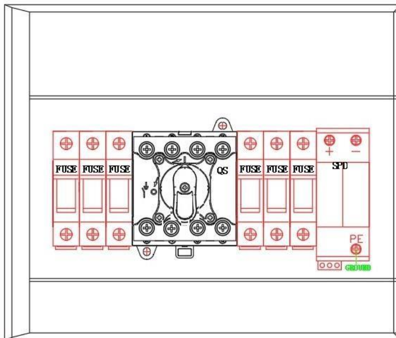
Рисунок 6.1 Выключатель PVBox в положении «ON».
