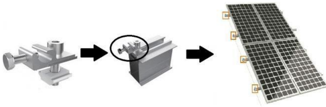
Рисунок 4.21 Установка зажима заземления.
