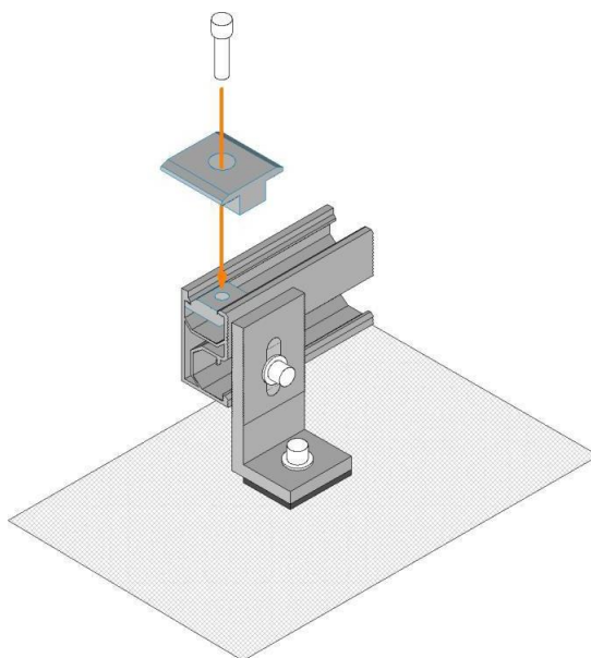
Рисунок 4.10 Установка универсального зажима.
