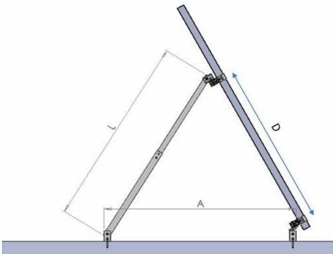
Рисунок 4.6 Параметры для установки оптимального угла.
