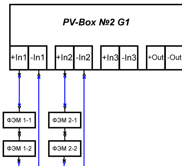
Рисунок 5.13 Структурная схема подключения фотоэлектрического модуля к PVBox.
