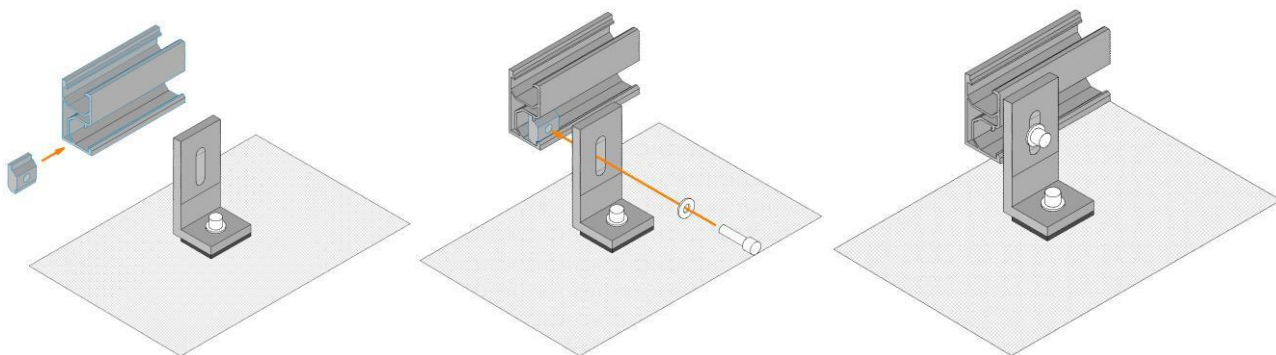
Рисунок 4.16 Соединение монтажного профиля и L-образного крепления.
