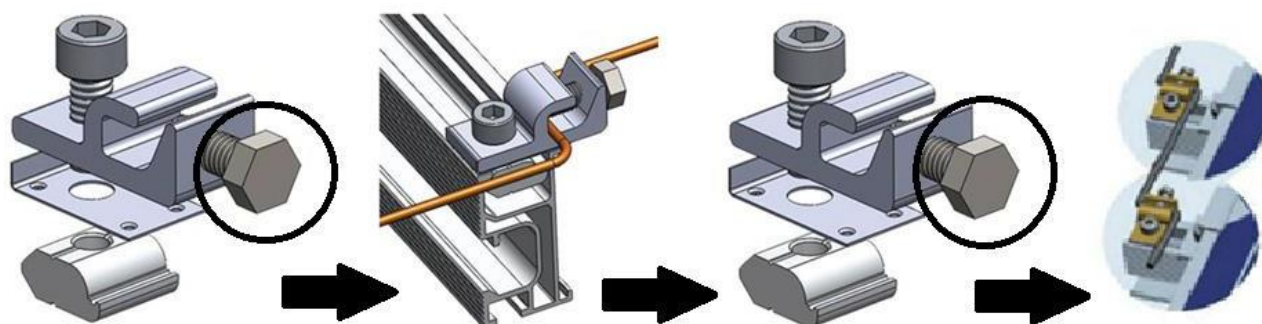
Рисунок 4.22 Установка кабеля заземления.
