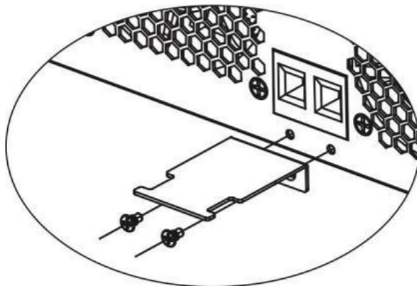
Рисунок 5.3 Установка вспомогательной пластины.
