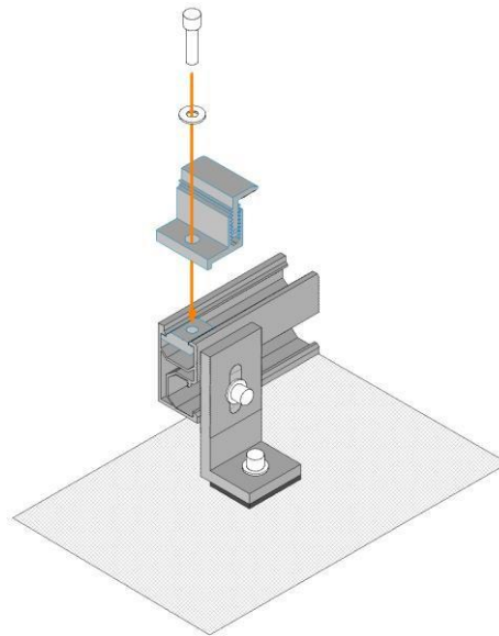
Рисунок 4.11 Установка регулируемого зажима.
