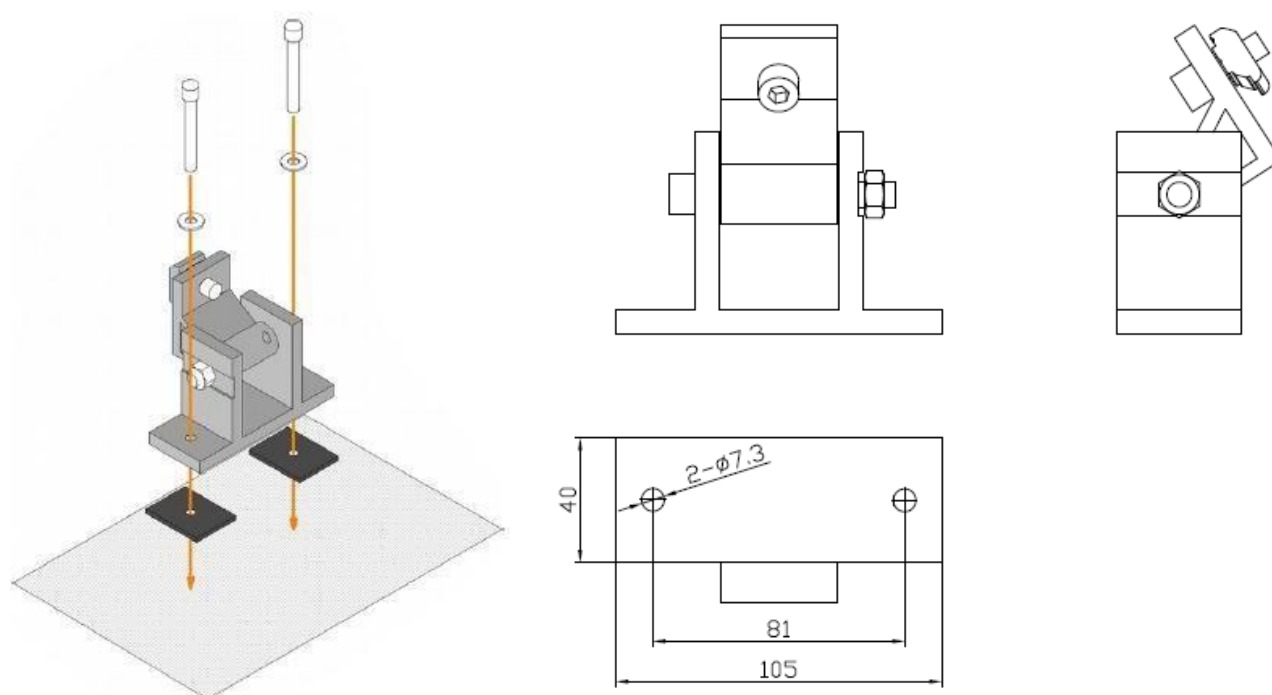
Рисунок 4.3 Монтаж передней стойки универсальной.
