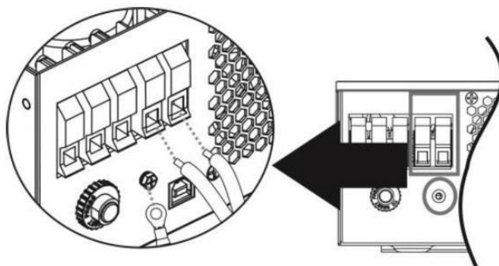
Рисунок 5.7 Подключение проводов выхода переменного тока к инвертору.
