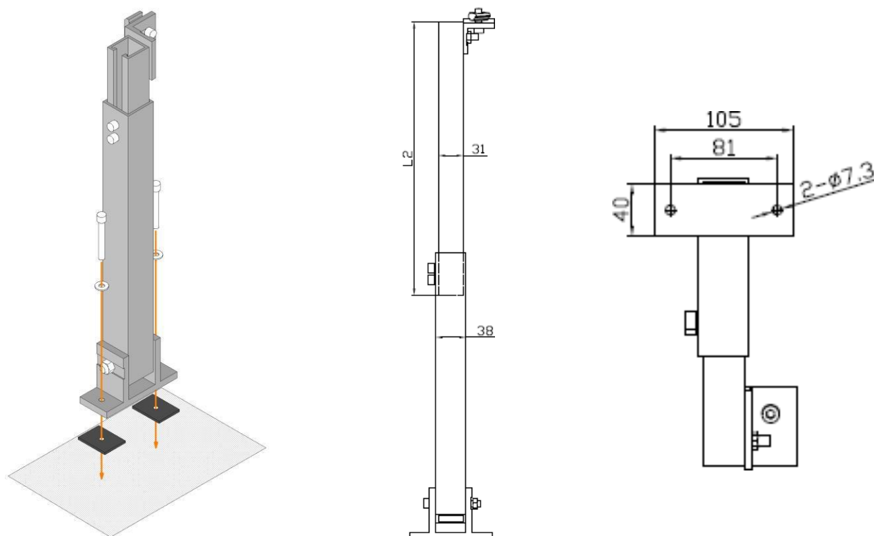
Рисунок 4.4 Монтаж задней стойки с регулируемым углом.
