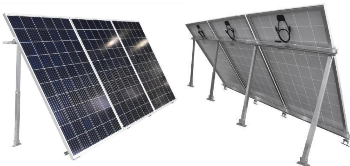
Рисунок 4.1 Массив ФЭМ «с углом» в сборе.
