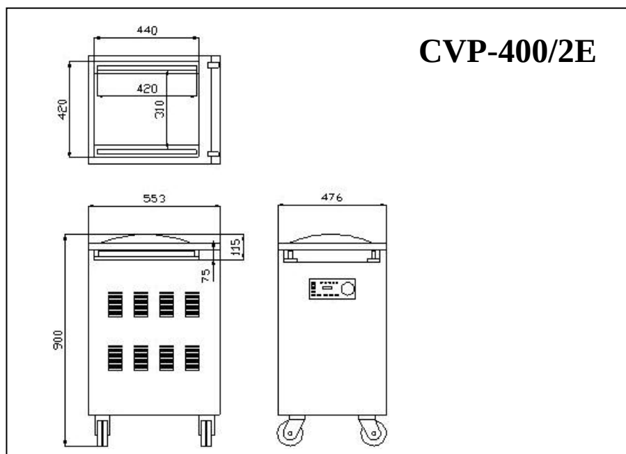
Рисунок 4.5 – Размеры вакуумного упаковщика модели CVP-400/2E
