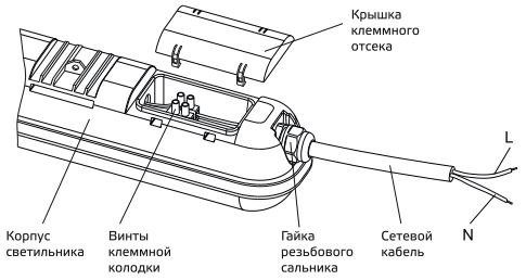
Рис. 1. Подключение светильников
