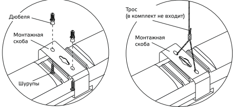
Рис. 2. Порядок монтажа
