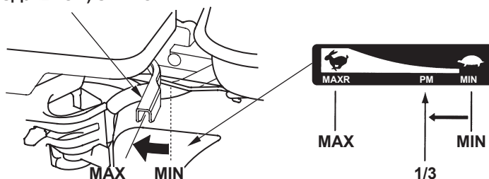
РЫЧАГ ДРОССЕЛЬНОЙ (ВОЗДУШНОЙ) ЗАСЛОНКИ
