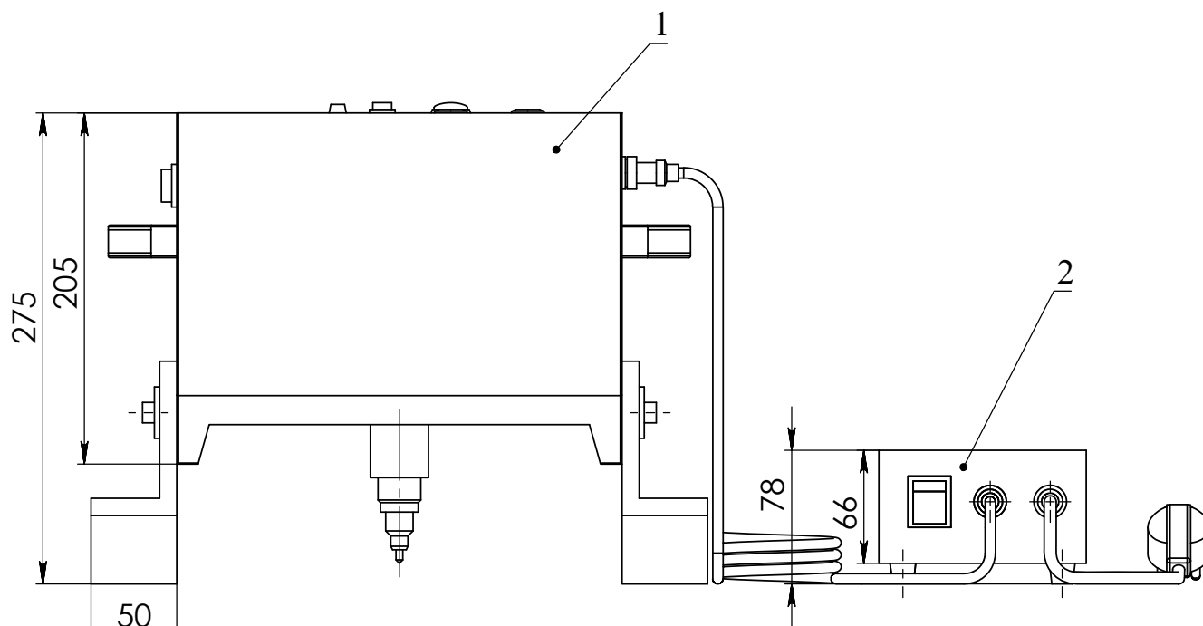
Рис. 1 Вид спереди 1 - Маркиратор 2 - Преобразователь напряжения
