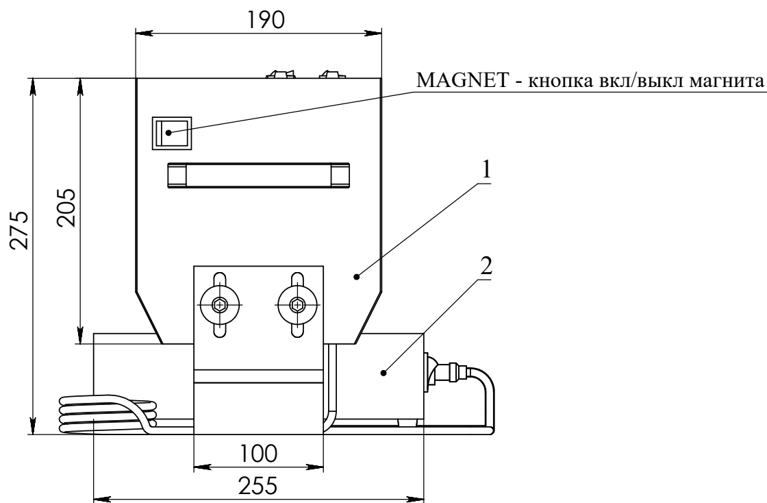
Рис. 3 Вид слева 1 - Маркиратор 2 - Преобразователь напряжения
