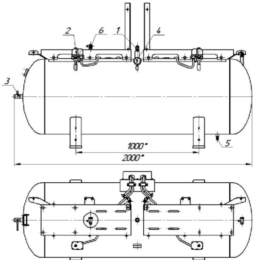
Рис.18. Ресивер установки компрессорной, модель К-30:
