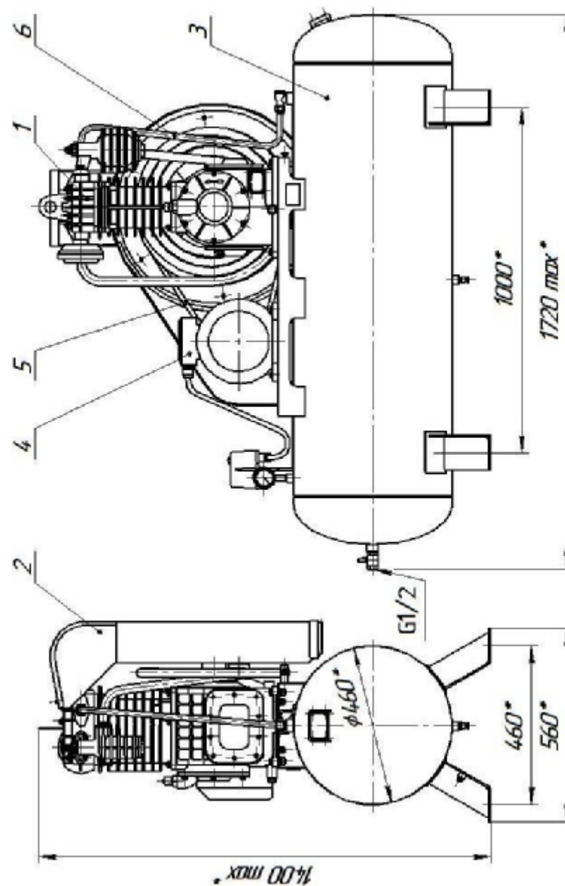
Рис. 5 Установка компрессорная, модель К-22:
