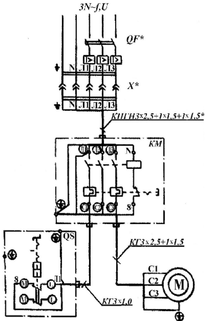
Рис.38. Схема электрическая принципиальная и соединений установок компрессорной, модель К-31
