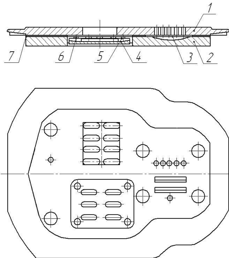
Рис.14. Блок клапанный:
