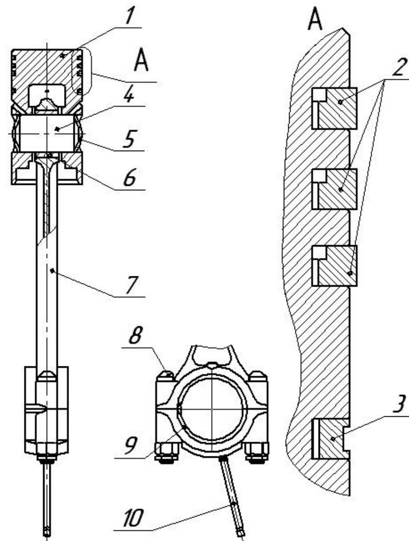
Рис.13. Поршень цилиндра высокого давления: 1-поршень; 2-кольцо компрессионное; 3- кольцо маслосъемное; 4-палец поршня; 5-заглушка; 6-втулка шатуна; 7-шатун; 8-болт шатунный; 9-вкладыш шатуна; 10-разбрызгиватель.
