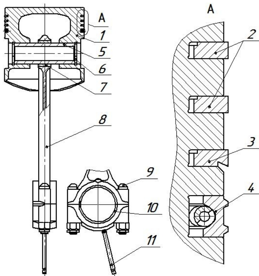
Рис.12. Поршень цилиндра низкого давления:
