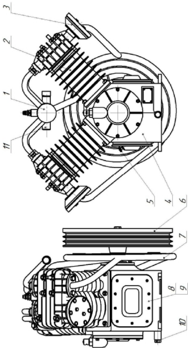
Рис. 10. Головка компрессорная С416М
