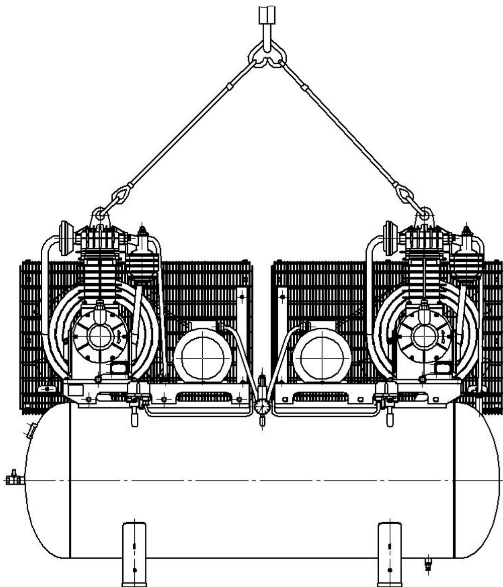
Рис.42. Схема строповки установки компрессорной мод. К-30.
