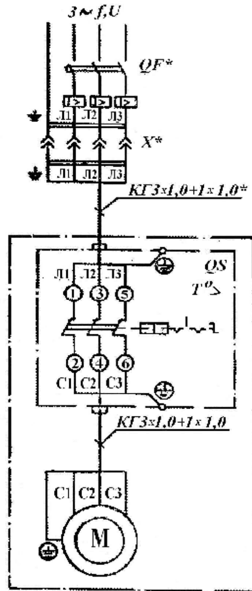
Рис.33. Схема электрическая принципиальная и соединений установки компрессорной, модель К-2.
