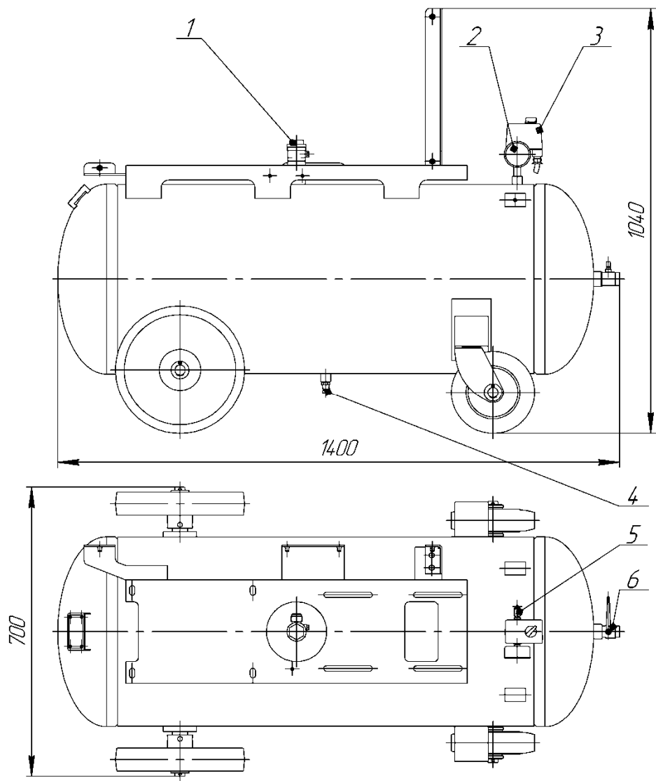
Рис.16. Ресивер установки компрессорной, модель К-31: 1-клапан обратный; 2-манометр контроля давления воздуха; 3-реле давления; 4-пробка сливная; 5- клапан предохранительный; 6- вентиль раздаточный.
