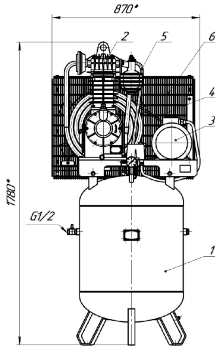
Рис. 7. Установка компрессорная, модель KB-15: 1-ресивер; 2-головка компрессорная; 3-двигатель; 4-приводные ремни; 5-трубопровод; 7-ограждение.
