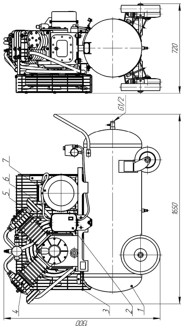
Рис. 8. Установка компрессорная, модель К-31: 1-ресивер; 2-пускатель магнитный; 3-ограждение; 4-головка компрессорная; 5- трубопровод; 6- ремни приводные; 7-двигатель.
