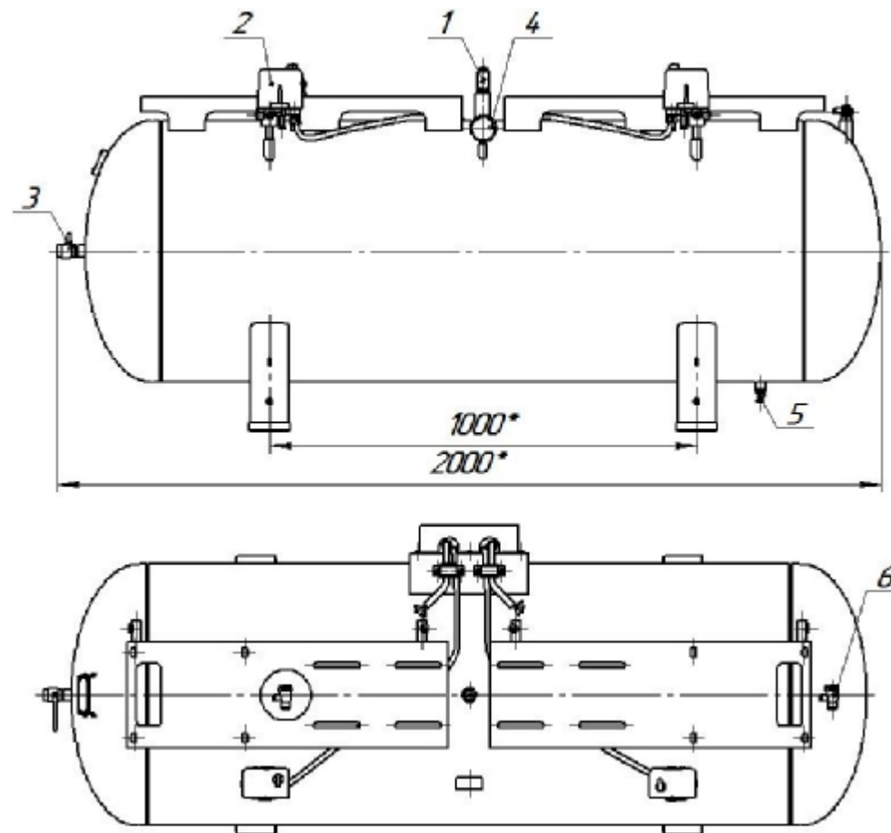
Рис.19. Ресивер установки компрессорной, модель К-20:
