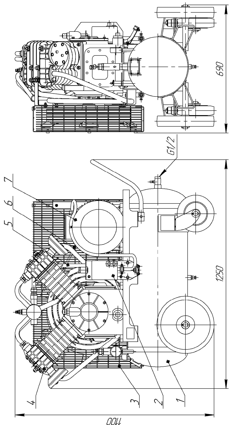
Рис. 6. Установка компрессорная, модель К-6:
