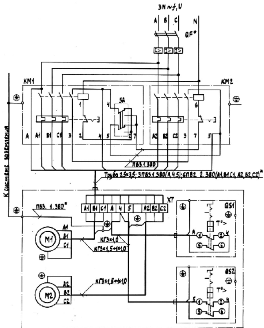
Рис.36. Схема электрическая принципиальная и соединений установки компрессорной, модель К-20 Схема электрическая принципиальная и соединений установки компрессорной, модель К-30 (различием является кабель от двигателей М1 и М2 до клеммного блока КГ 3×1,0+1×1,0).
