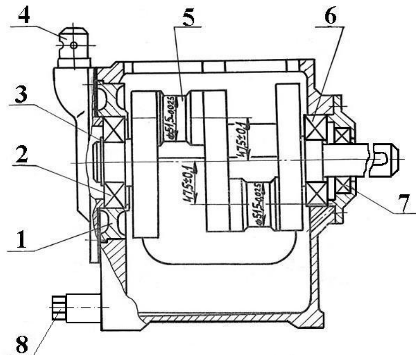
Рис.11. Картер:
