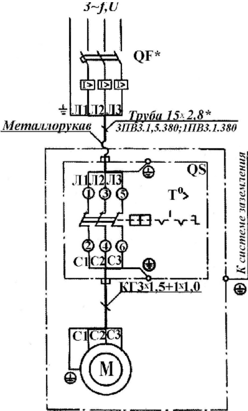
Рис.37. Схема электрическая принципиальная и соединений установки компрессорной, модель К-22
