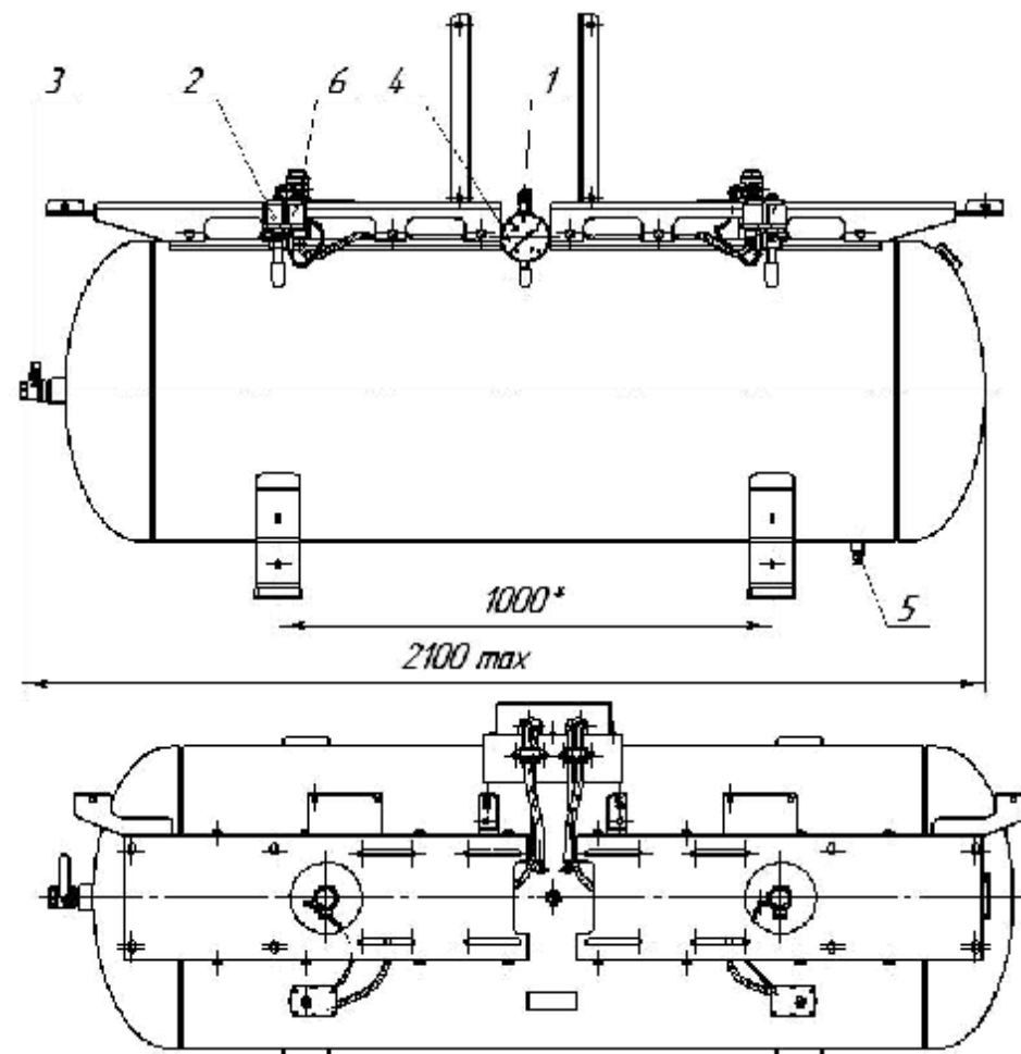
Рис.17. Ресивер установки компрессорной, модель К-3: 1-клапан предохранительный; 2-реле давления; 3-вентиль раздаточный; 4-манометр контроля давления воздуха; 5-пробка сливная; 6-клапан обратный.
