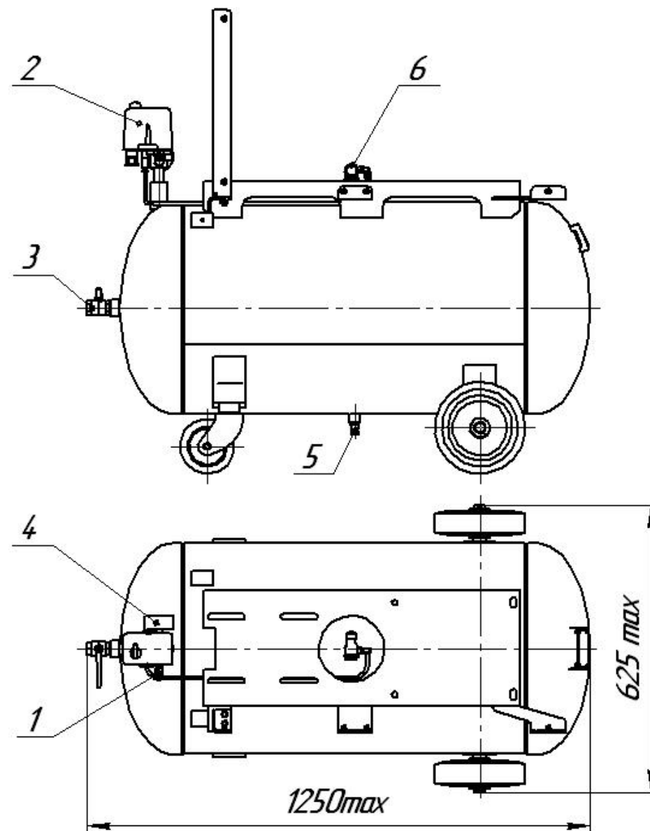
Рис.15. Ресивер установки компрессорной, модель К-2: 1-клапан предохранительный; 2-реле давления; 3-вентиль раздаточный; 4-манометр контроля давления воздуха; 5-пробка сливная; 6-клапан обратный.
