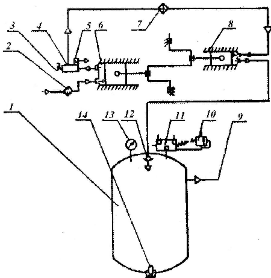
Рис.28. Схема пневматическая принципиальная установки компрессорной, модель KB-15:
