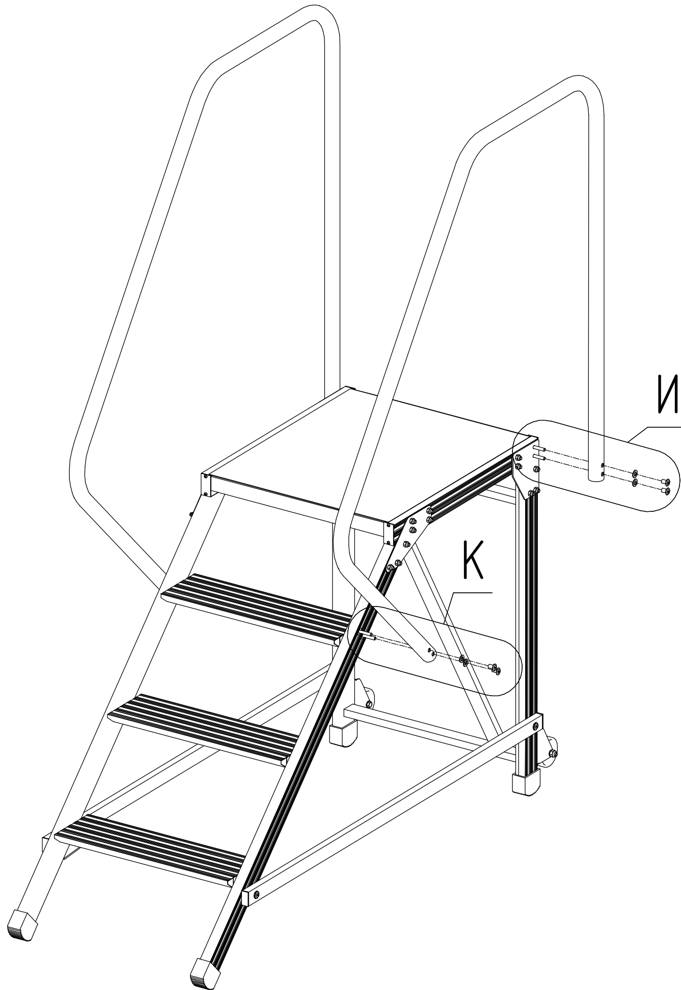
Рисунок 5 – Установка поручней.
