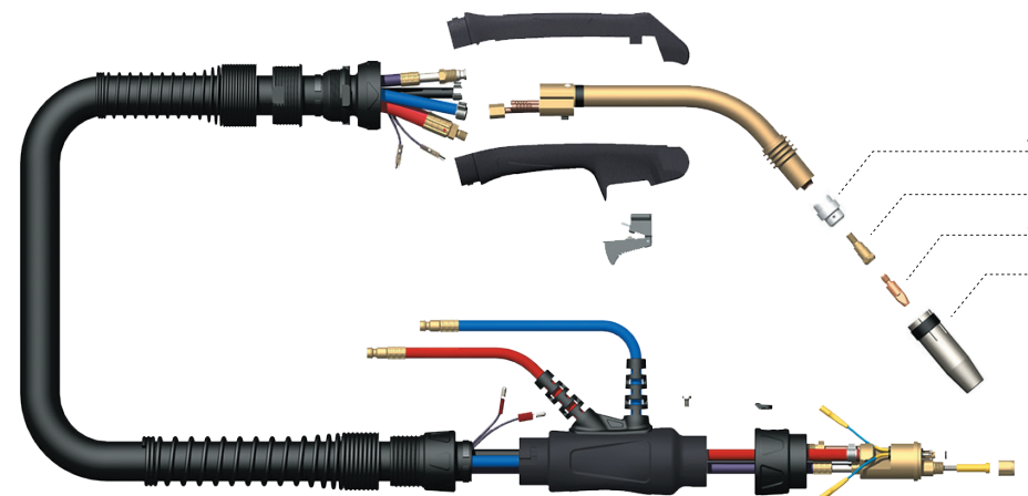
1. Газовое сопло (L=63,5)
