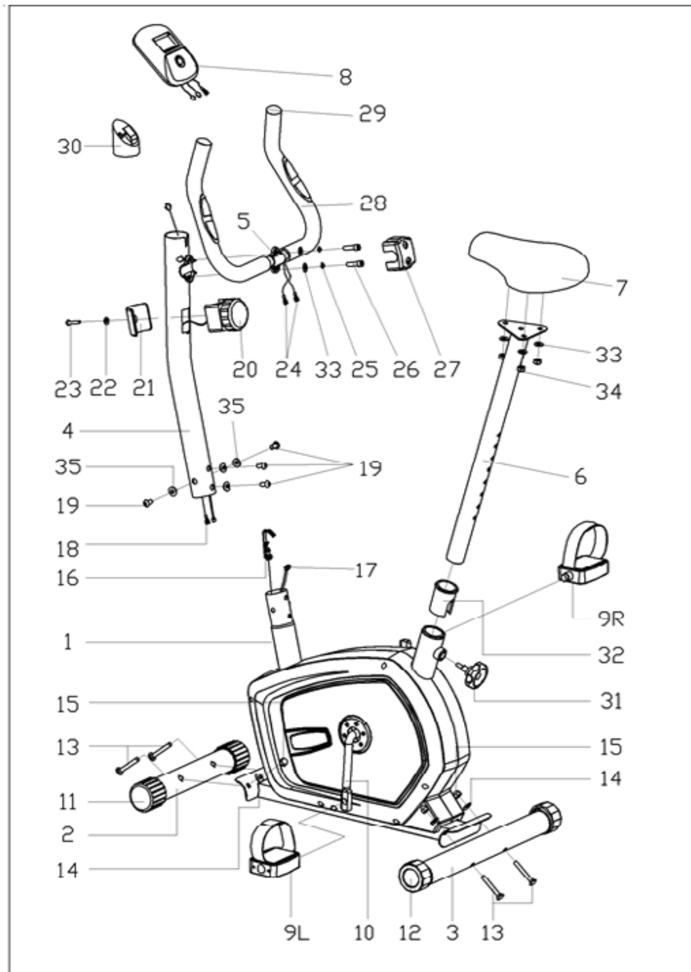
РИСУНОК-СХЕМА
