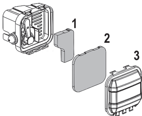
Рис. 10 Воздушный фильтр
