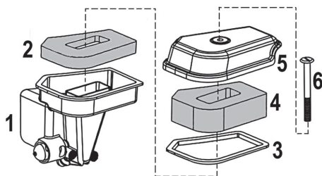
Рис. 9 Воздушный фильтр
