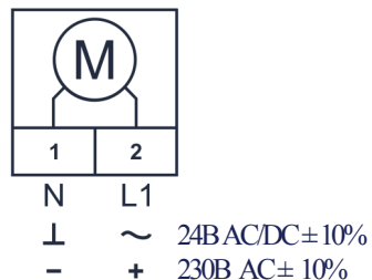
Привод SC-05D...
