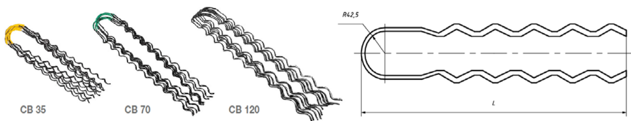
Рис. 1. Внешний вид спиральных вязок типа СВ.
