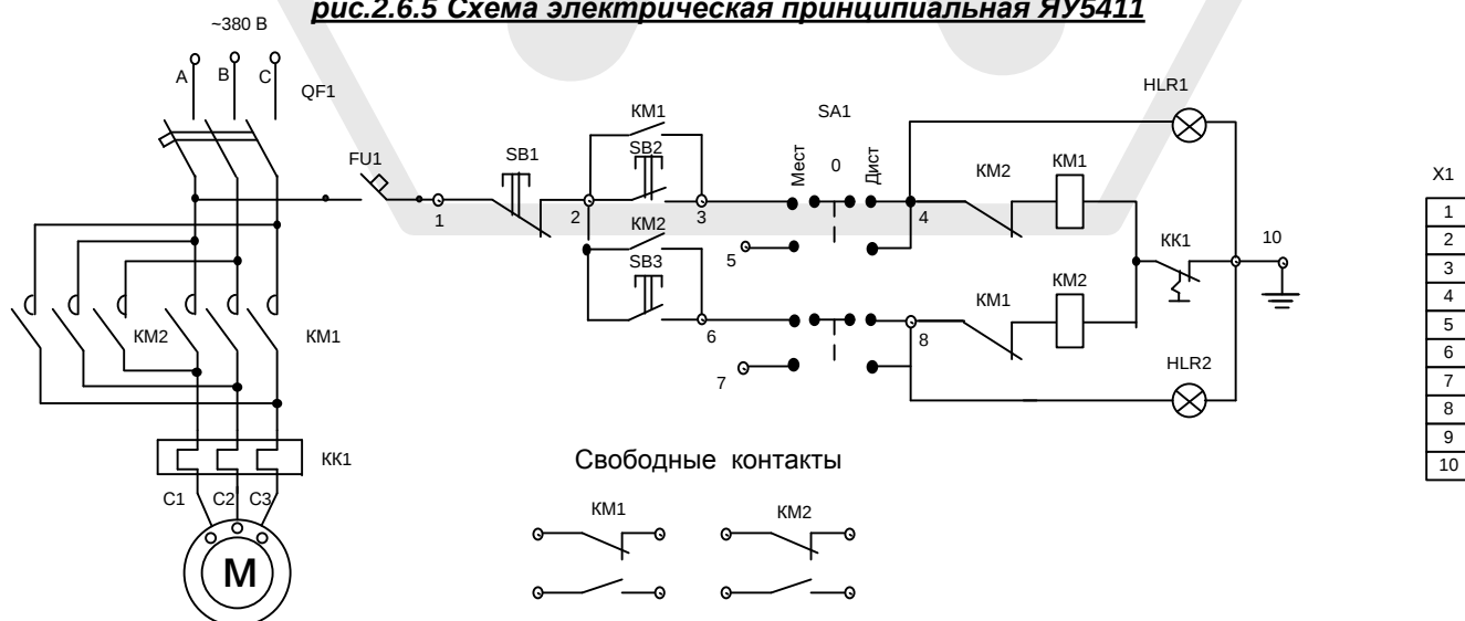
рис.2.6.5 Схема электрическая принципиальная ЯУ5411
