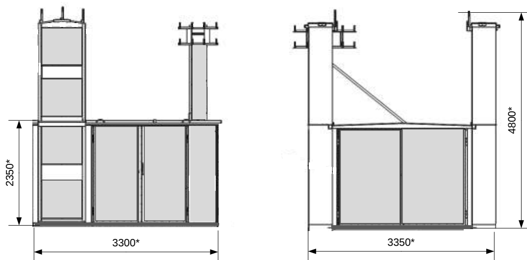
КТП проходного типа . Исполнение воздух-воздух
