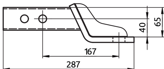
00045502 Кронштейн 50x50 для фаркопа усиленный
