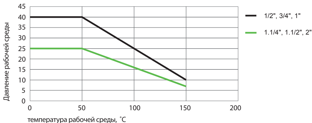
График зависимости давления от температуры
