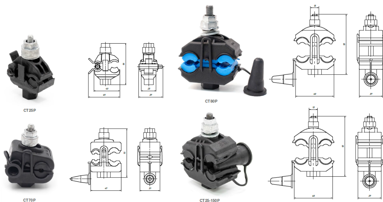
Рис. 1. Внешний вид герметичных ответвительных зажимов типа СТ.
