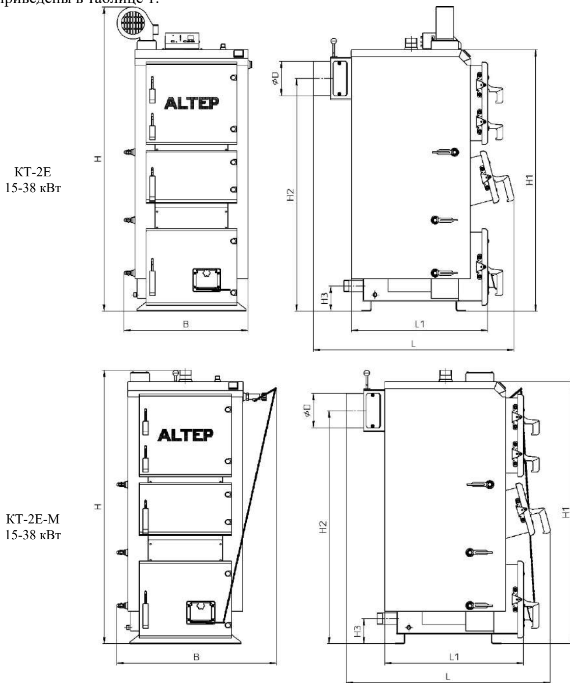
Рисунок 1 – Габаритный чертеж котла типа КТ-2Е (КТ-2Е-М)
