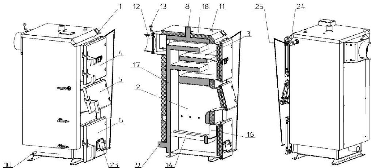
Рисунок 2 – Внешний вид и основные элементы котла
