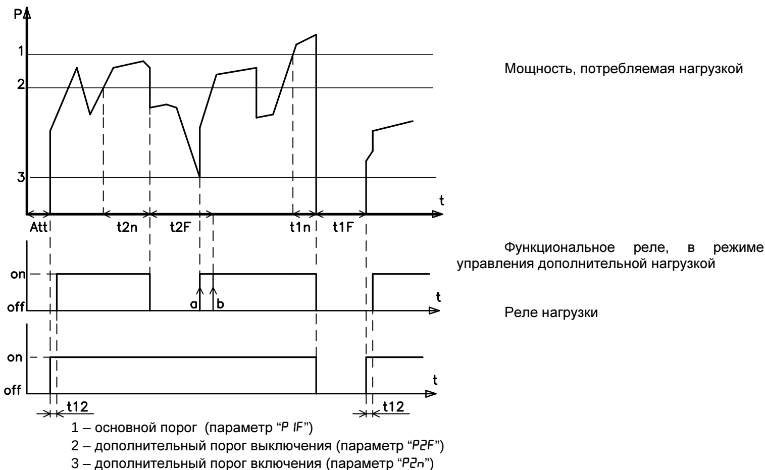
Рисунок 1.3 - Работа ОМ-310 в режиме ограничения мощности при rS=2
