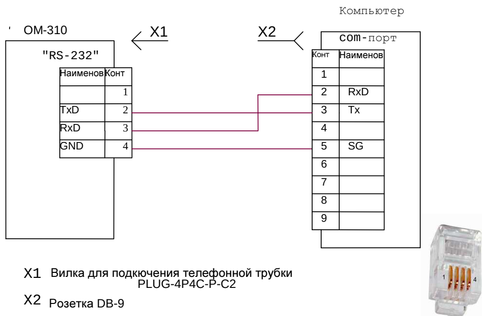
Рисунок 2.3 - Схема подключения ОМ-310 к компьютеру
