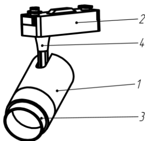
Рисунок 2 — Конструкция светильника.
