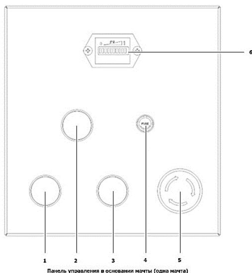
Панель управления в основании мачты (одна мачта)
