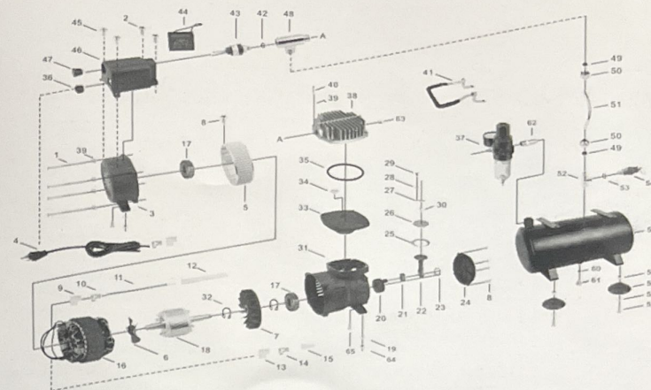
СПИСОК ДЕТАЛЕЙ КОМПРЕССОРА TNT-AIR AS-326
