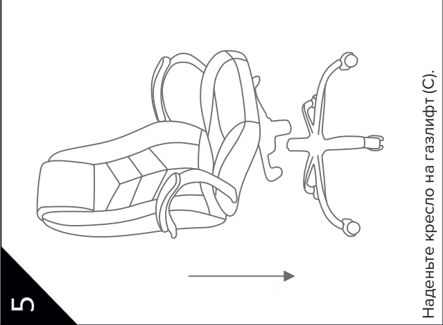
Подлокотники (F) прикрепите к спинке (G) и сиденью (Н) с помощью винтов (L).
