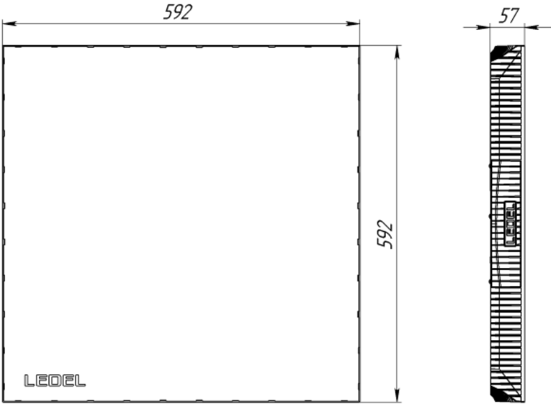
Рисунок 1 Светильник «L-office 32 Standart», «L-office 55 Standart»
