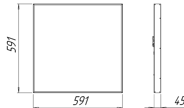
Рисунок 1 Светильник «L-office 32 Standart/Em», «L-office 55 Standart/Em»
