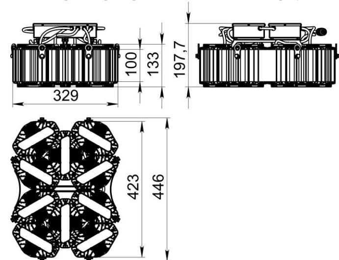
Рисунок 1 Светильник «L-lego II 500» с подвесным креплением.
