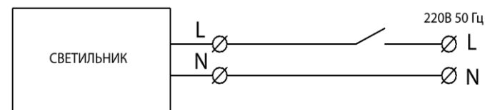
Рисунок 2 Схема подключения светильника
