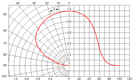
Рисунок 3 Тип КСС в исполнении «Д»
