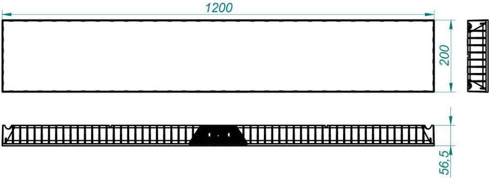
Рисунок 1б Светильник «L-school 32 Standart», «L-school 55 Standart»
