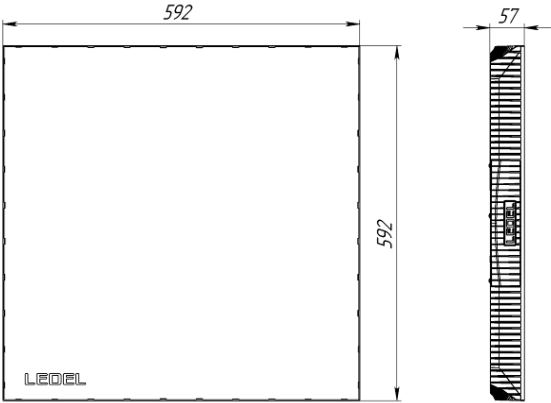
Рисунок 1 Светильник «L-office 32 S Premium»
