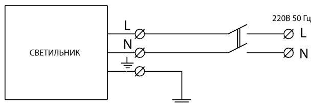
Рисунок 2 Схема подключения светильника «L-office 32»
