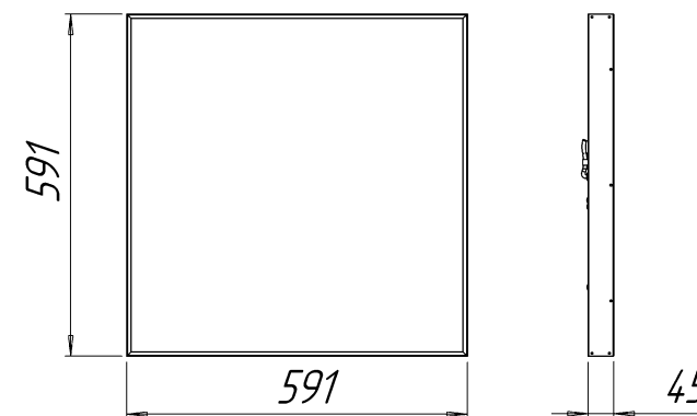
Рисунок 1 Светильник «L-office 32 Premium/Em»
