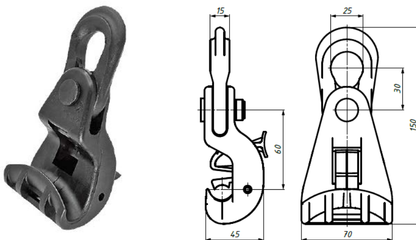
Рис. 1. Внешний вид поддерживающих зажимов PS 1500, PS 2000.
