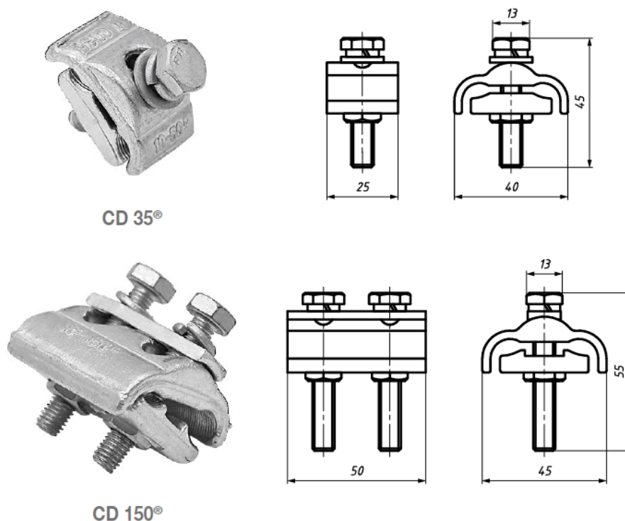
Рис. 1. Внешний вид плашечных зажимов CD 35, CD 150.
