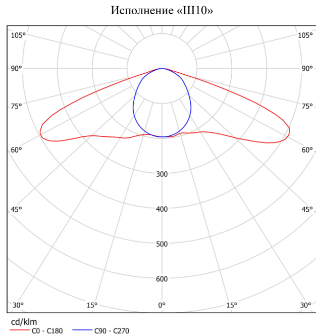
Рисунок 3 Типы КСС
