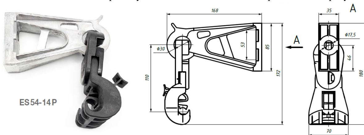
Рис. 1. Внешний вид комплекта промежуточной подвески ES 54-14 Р.
