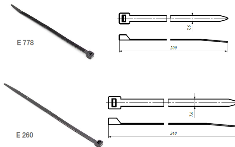
Рис. 1. Внешний вид стяжных ремешков Е 778, Е 260.
