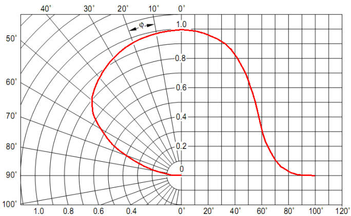
Рисунок 3 Тип КСС в исполнении «Д»
