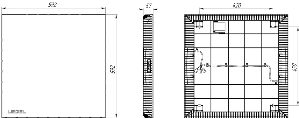
Рисунок 1 Светильник «L-office 32/Em»
