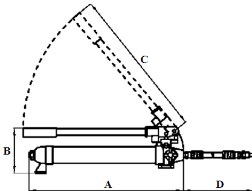
Рисунок 3. Размеры насоса.
