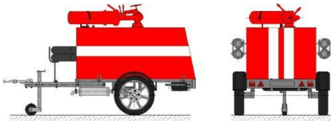
Рис. 1 Мотопомпа МП-40/100.1 Общий вид
