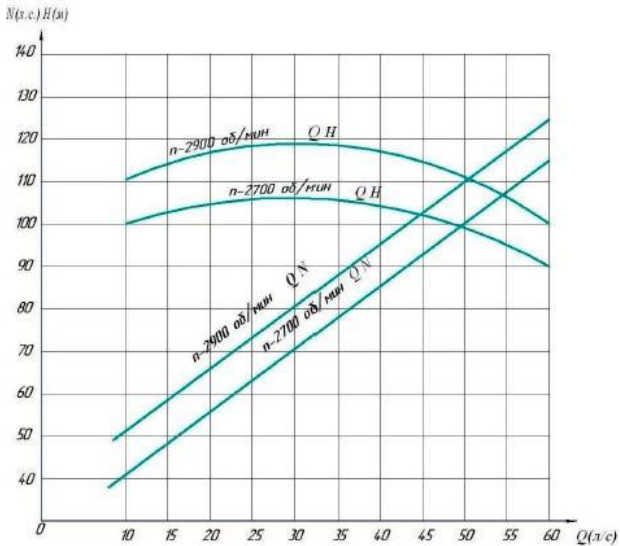
Напорная характеристика МП-40/100.1
