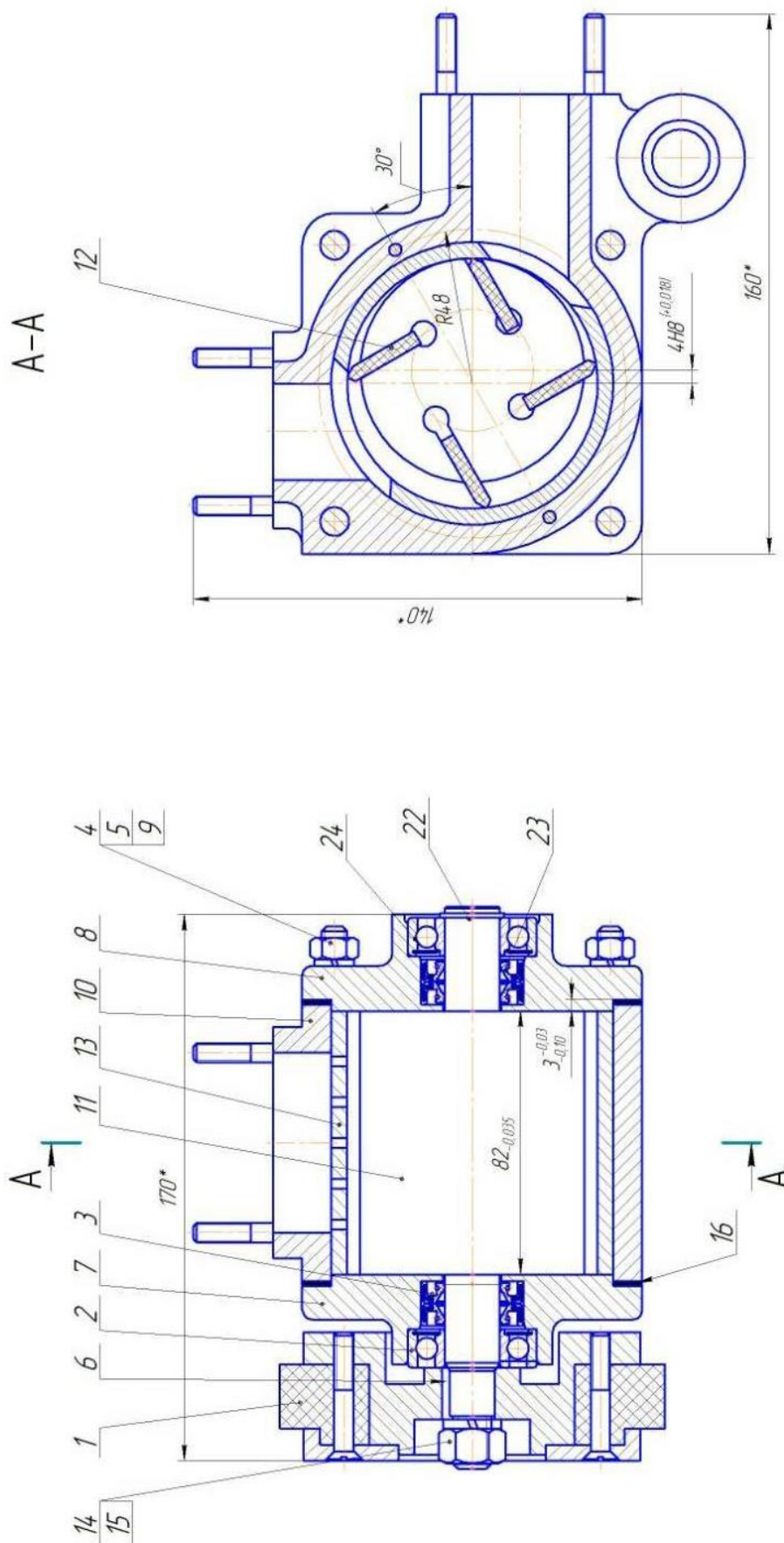
Рис. 5 Вакуумный насос
