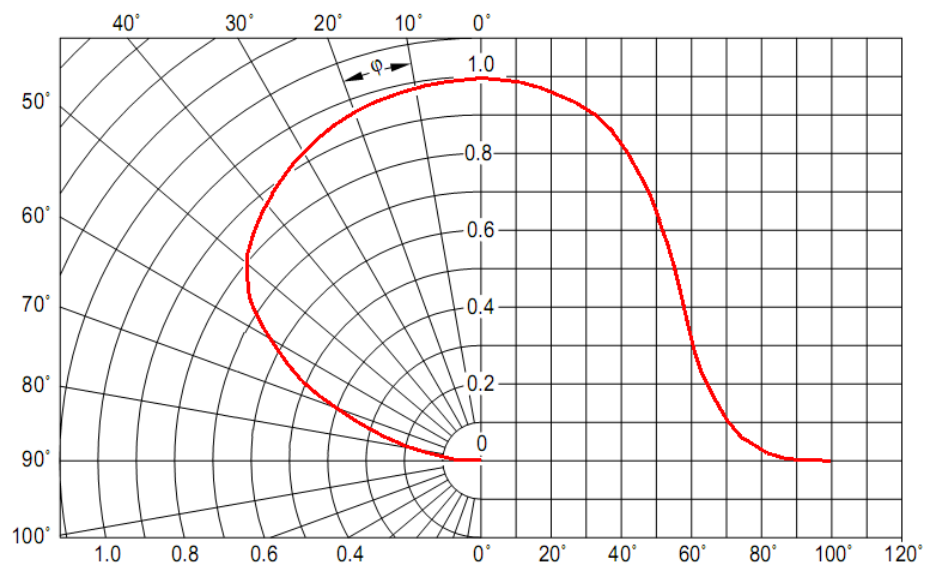
Рисунок 3 Тип КСС в исполнении «Д»
