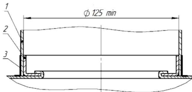
Рисунок 8. Схема подсоединения газоотводящей трубы
