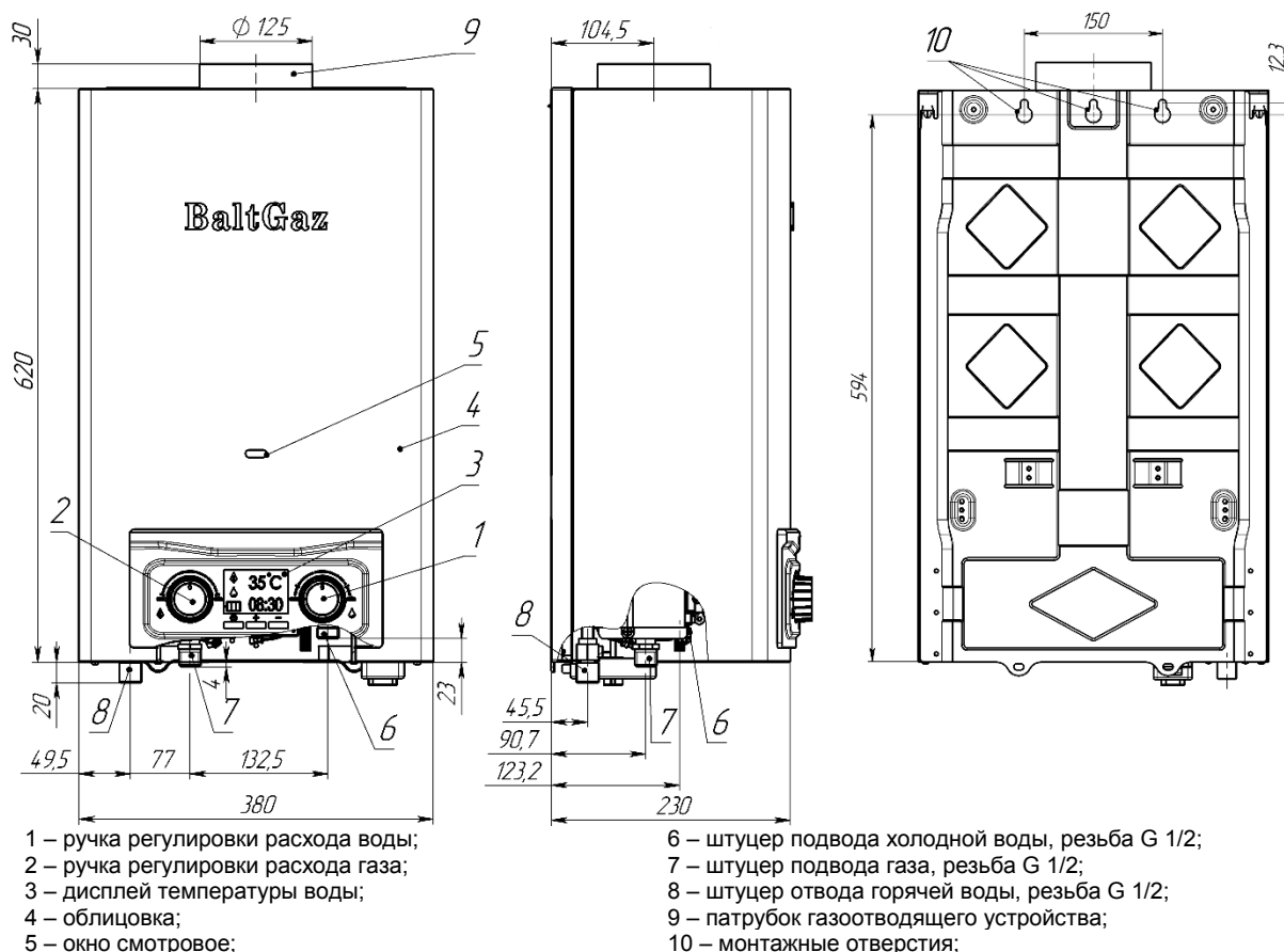
Рисунок 1. Габаритные и присоединительные размеры аппарата
